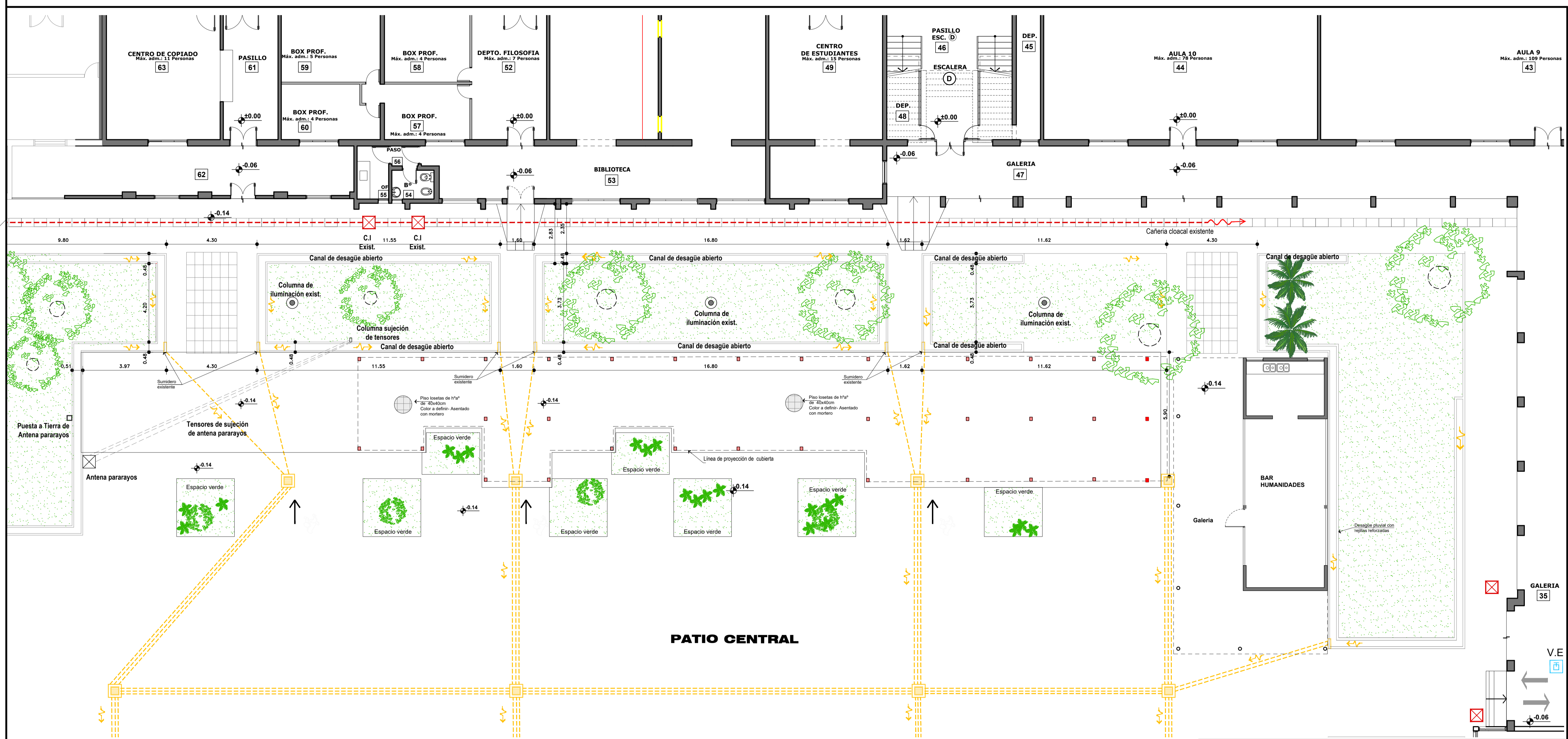
PLANTA DE DESAGÜES PLUVIALES - SECTOR PATIO CENTRAL - FAC. HUMANIDADES ESC 1:100
